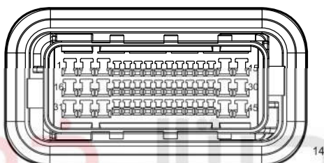
I_BFRD Body W.H. Connector Connecting FL Door W.H.
