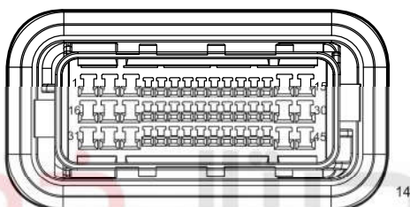
I_BFRD Body W.H. Connector Connecting FR Door W.H.
