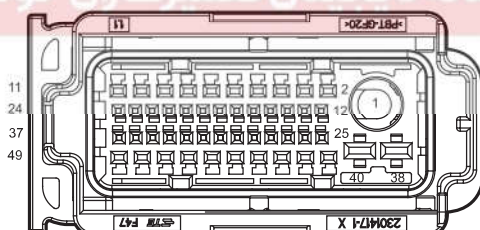
I_FRDB FR Door W.H. Connector Connecting Body W.H.
