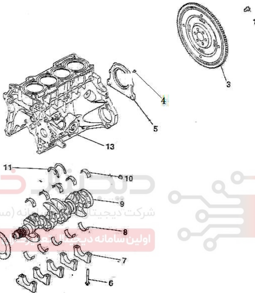
مجموعه بلوک سیلندر
