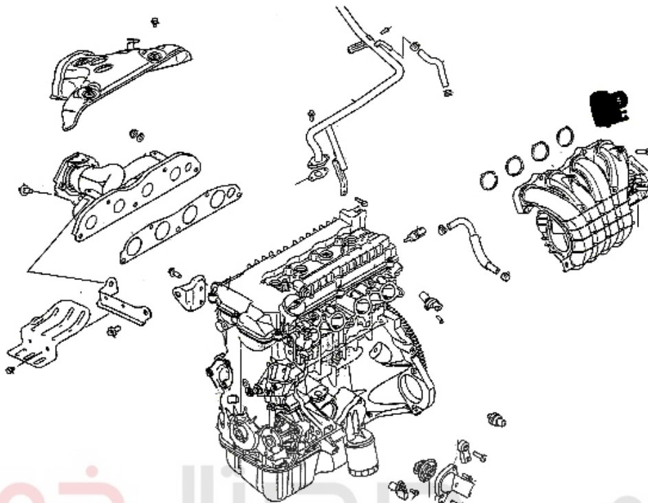
دیاگرام منیفولد هوا و منیفولد دود
