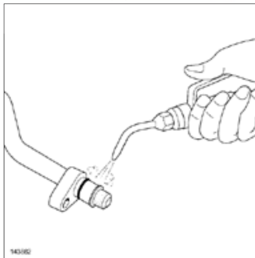
با استفاده از نازل هوای فشرده بر روی سطح و واشرهای لوله‌های اتصال بدمید. سطح و واشرهای لوله‌های اتصال را با روغن تهویه مطبوع روانکاری کنید (به 62A، تهویه مطبوع، تهویه مطبوع، قطعات و مواد مصرفی برای تعمیرات رجوع کنید). درپوش‌های مسدود کننده را بردارید.
