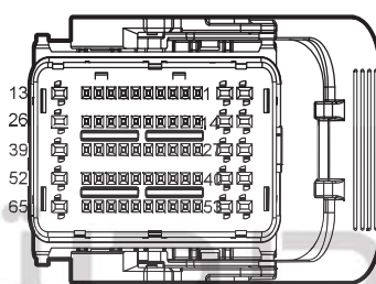
E19 UAES QNUEmission VI
